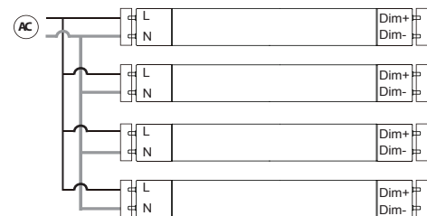
Fig:4 - Multiple lamps wiring
