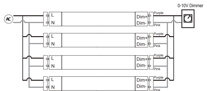
Fig:4 - Multiple lamps wiring
